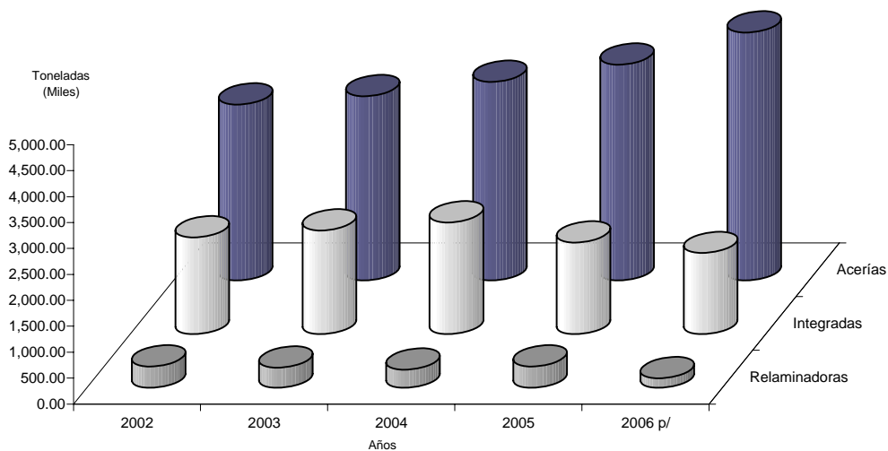
Producción de Productos Siderúrgicos No Planos
