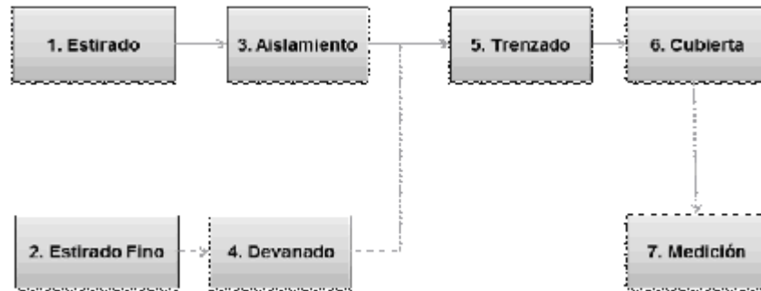
Diagrama 1. Proceso de producción de cable coaxial
