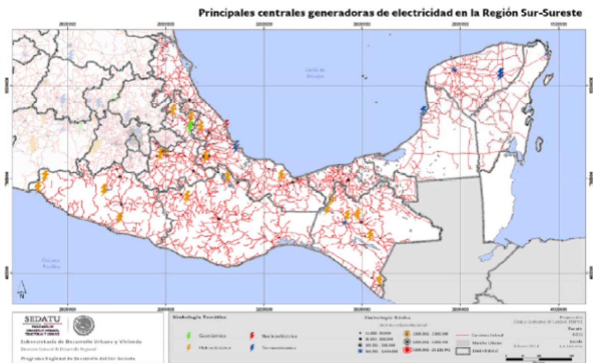
Mapa 26. Principales centrales generadoras de electricidad
