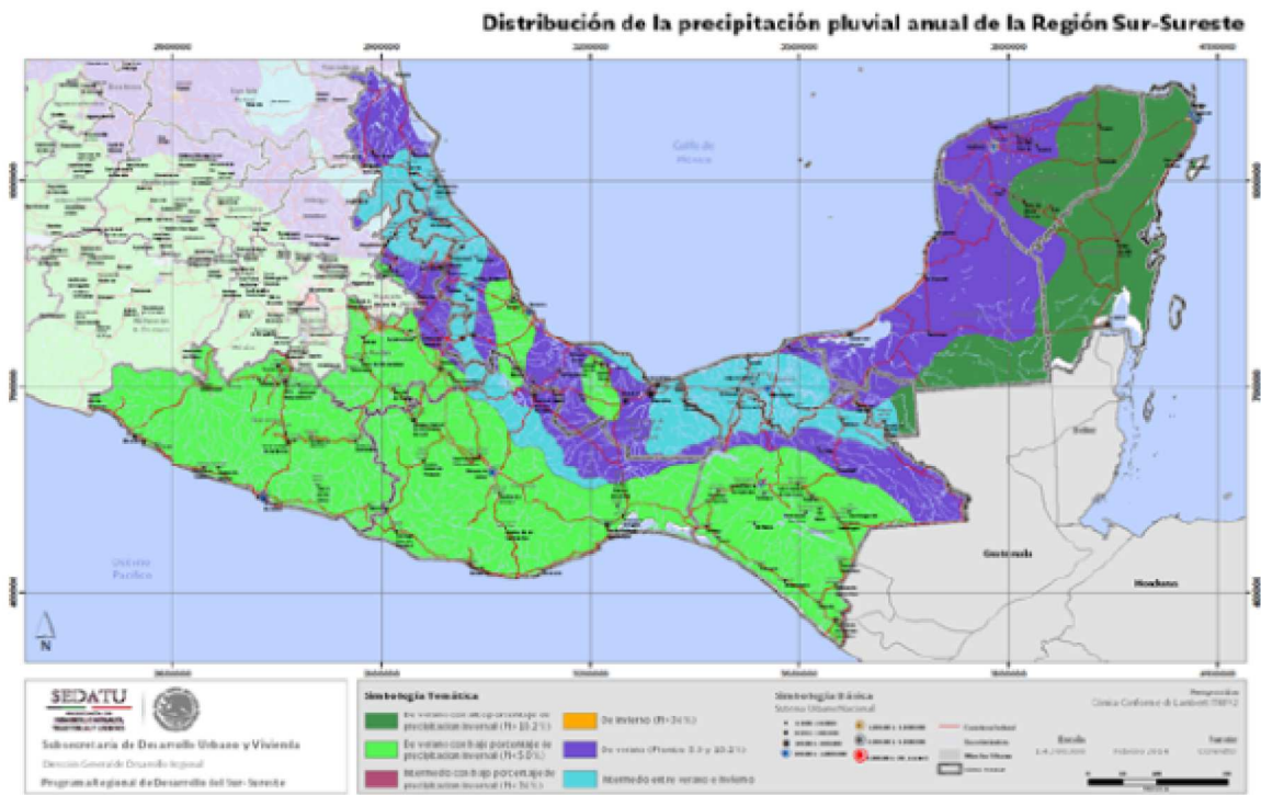
Mapa 5. Distribución de la precipitación anual
